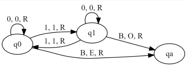
图灵机状态转移图
